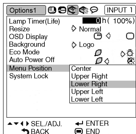
Sub menu
