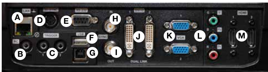
图 4-7. 连接器面板
